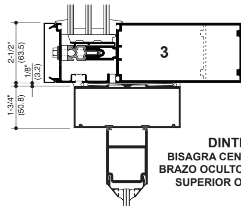
DINTEL CERRADOR CON BRAZO DE DESPLAZAMIENTO DE ACCIÓN SENCILLA
