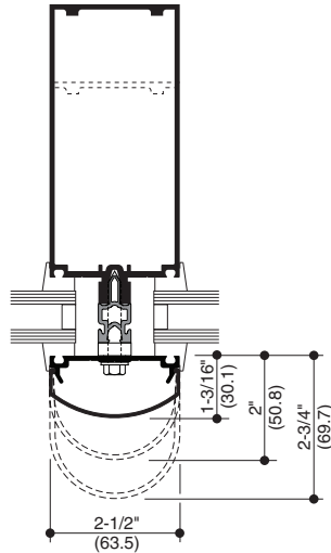
OPCIONAL CUBIERTAS DE BORDE REDONDEADO
