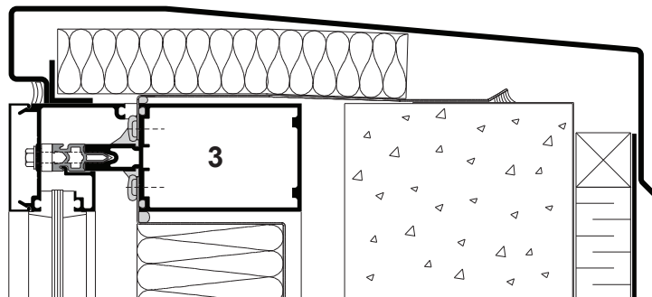
TRAVESAÑO SUPERIOR A RAS DEL ANTEPECHO
