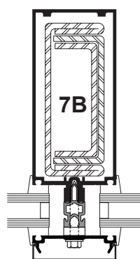
ACERO DE REFUERZO SEGÚN SE REQUIERA
