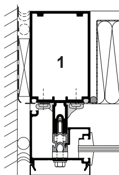
PARTELUZ DE JAMBA EN ANTEPECHO (Con unión de barrera de vapor)
