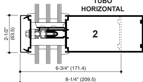
DORSO ABIERTO HORIZONTAL
