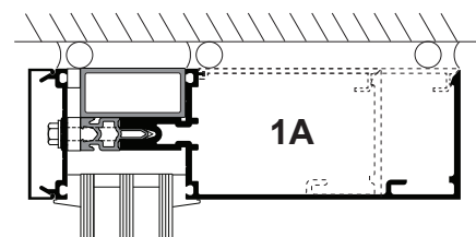
TUBO HORIZONTAL
