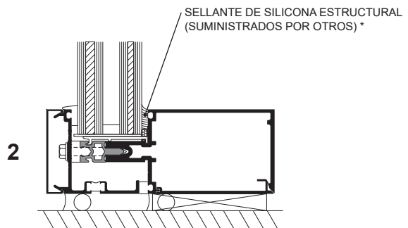
ALFÉIZAR
