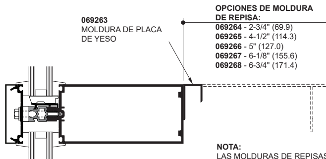
MOLDURA DE REPISA INTERIOR
